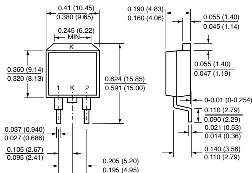
TO-263AB
