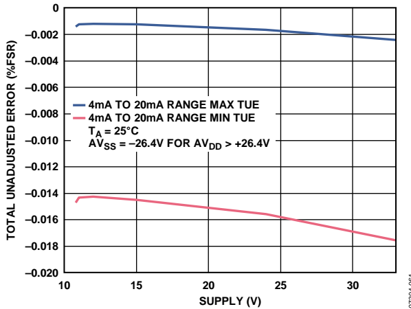
Figure 46. Total Unadjusted Error vs. AV DD , Internal R SET
