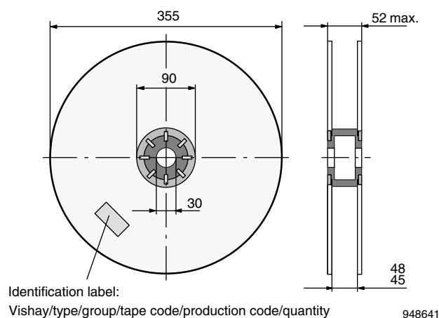
Fig. 16 - Reel Dimensions
