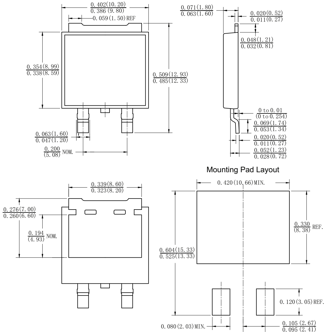
TO-263AC (SMPD)
