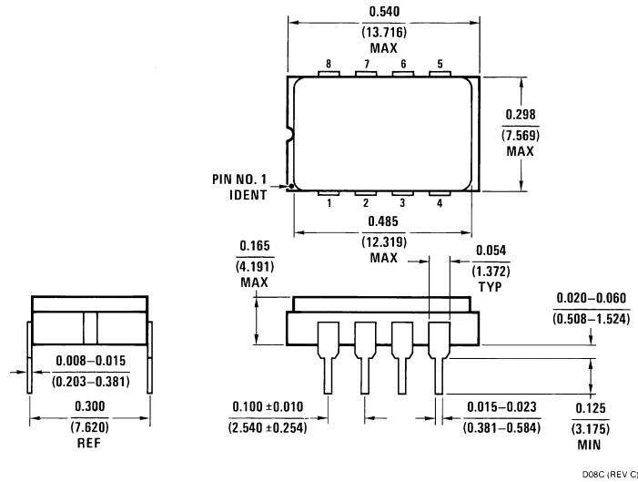
Hermetic Dual-In-Line Pkg. (D) Order Number LMC662AMD NS Package Number D08C
