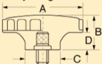
Projecting Stud
