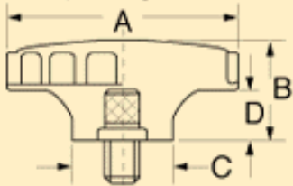
Projecting Stud
