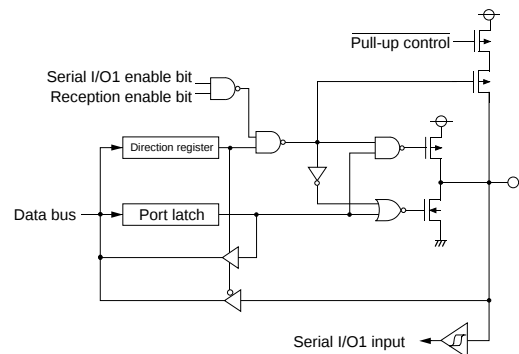
(8)Port P46
