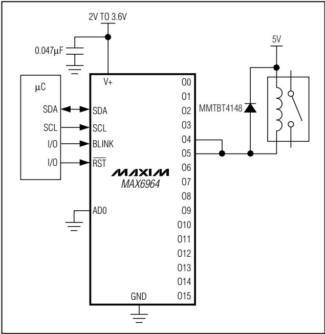
그림 19. 인덕티브 부하의 다이오드 보호 스위칭
