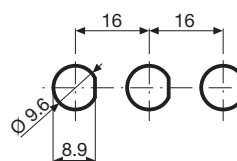
Cut-out Montageöffnung
