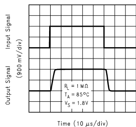
Time (10 \mu s /div) DS100979-F6
