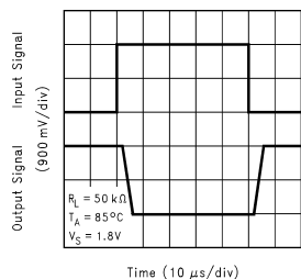
Time (10 \mu s /div) DS100979-D7
