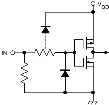
Dwg. EP-010-4A
