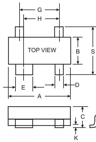
SOT-343 / SOT-143
