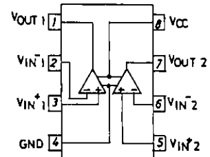
LA6358N
