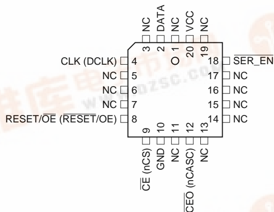
20-Pin PLCC
