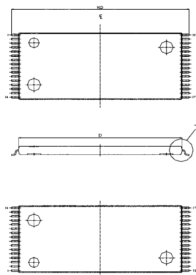
TSOP - 32
