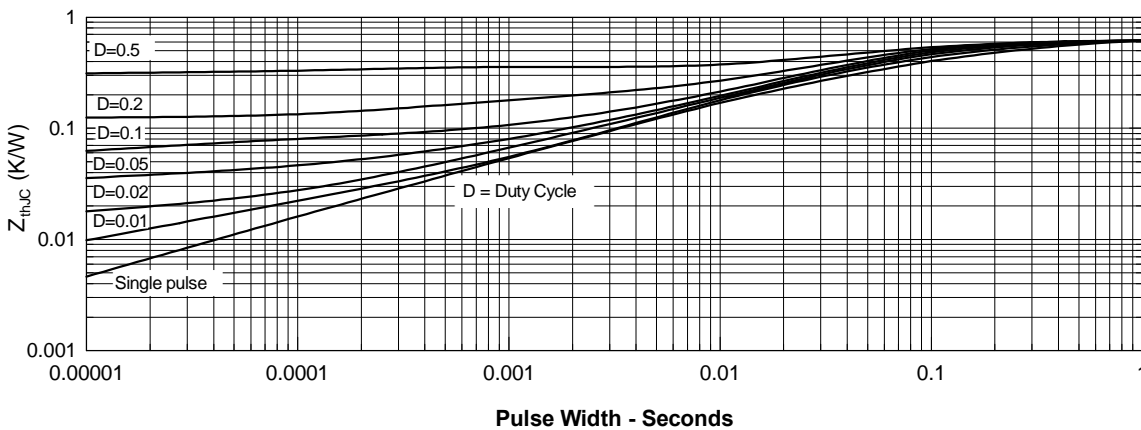
Fig. 10. Thermal Impedance
