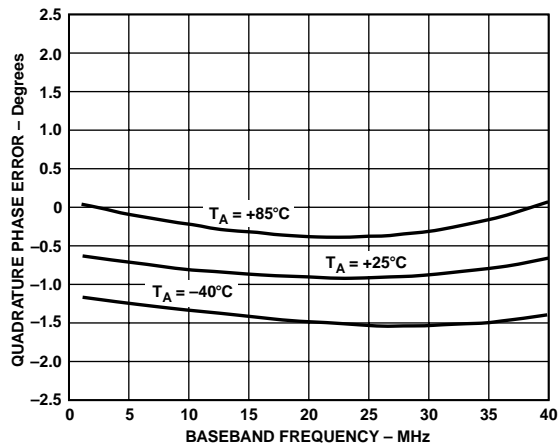
TPC 24. Quadrature Phase Error vs. F_{BB} , V_{GIN} = 0.7 V, V_S = 5 V
