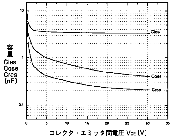
容量-コレクタ・エミッタ間電圧特性 ( T_j = 25^\circ\text{C} ) <INV部> Capacitance vs. Collector-Emitter voltage <INV>
