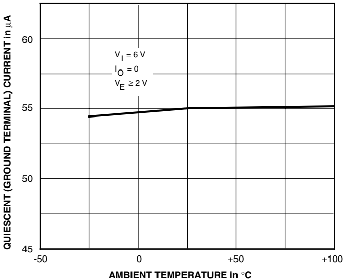
Dwg. GP-051-3
