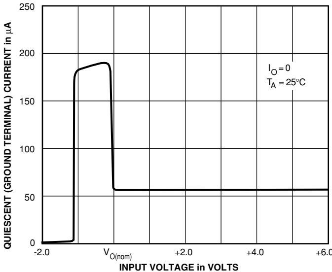
Dwg. GP-058-1
