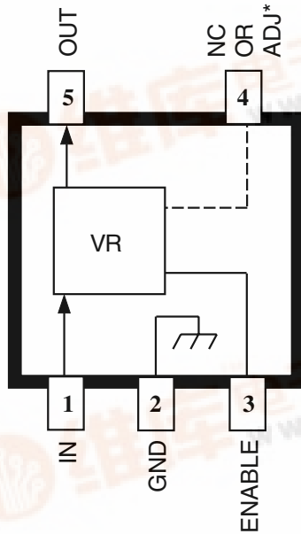
Dwg. PS-021-5
