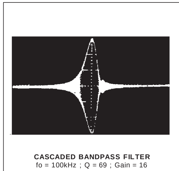
OUTPUT B
