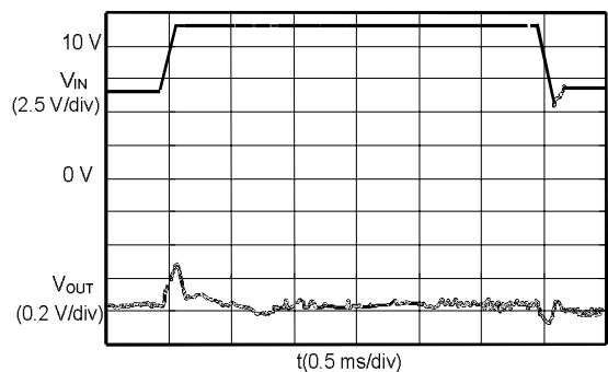
S-8520/1E33MC ( I_{OUT} :10 mA)
