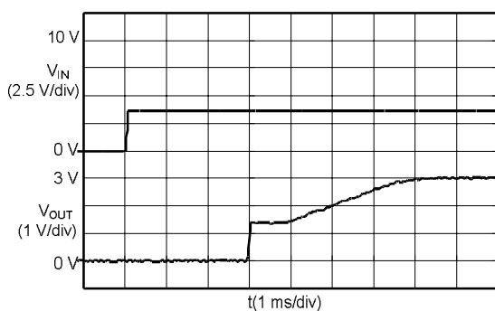
S-8520/1A30MC ( V_{IN} : 0 \rightarrow 3.6 V)
