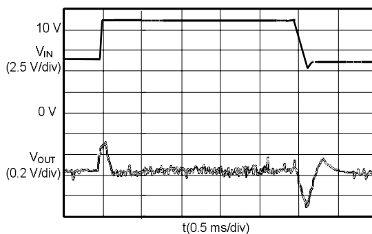
S-8520/1E33MC ( I_{OUT} :500 mA)
