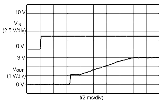
S-8520/1C30MC ( V_{IN} : 0 \rightarrow 3.6 V)
