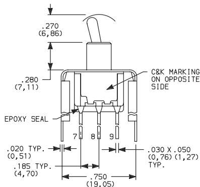
7301MD9_BE 3PDT
