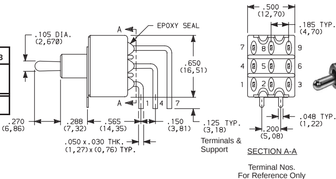
7301MD9ABE Horizontal Actuation 3PDT
