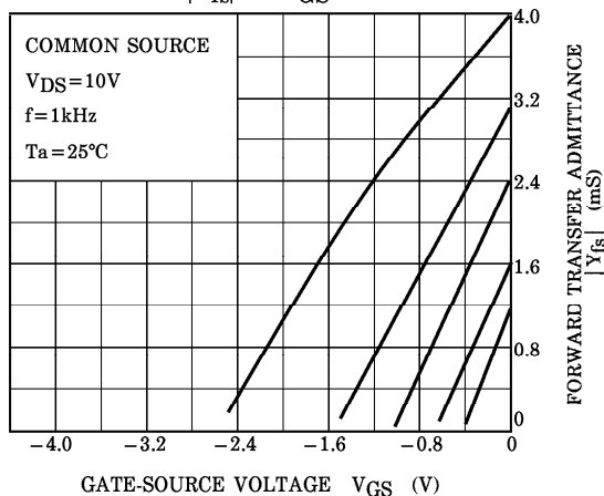
|Y_{fs}| - V_{GS}
