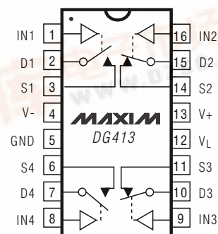
DIP/SO/TSSOP
