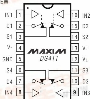
DIP/SO/TSSOP
