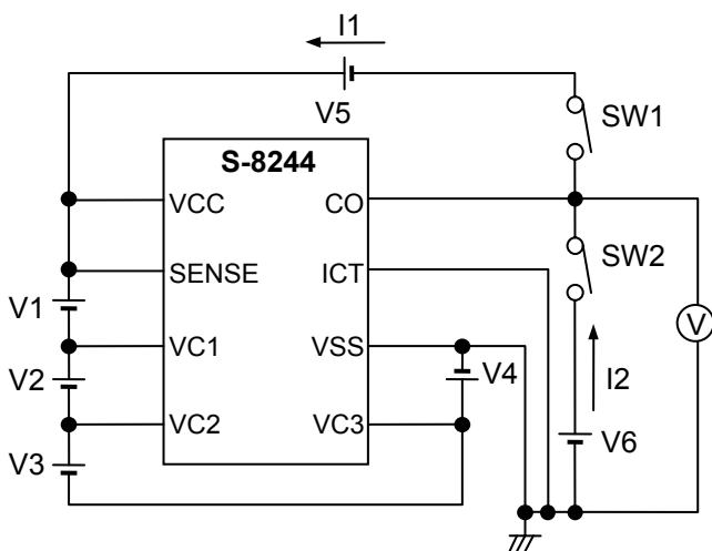
测定电路4
