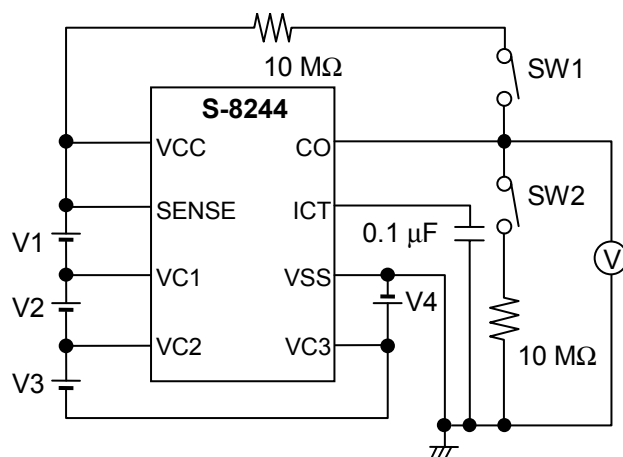
测定电路2
