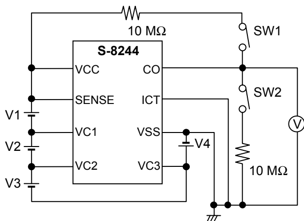
测定电路1
