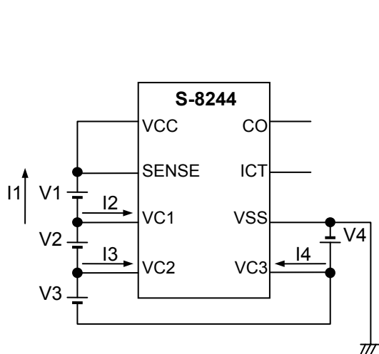
测定电路3
