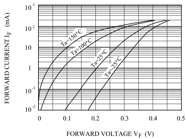
I_F - V_F
