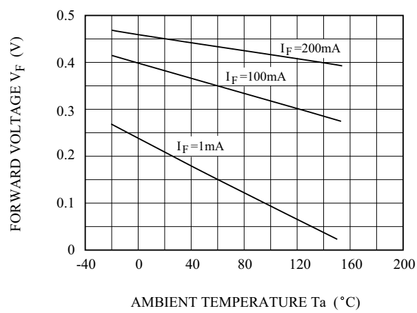
V_F - T_a
