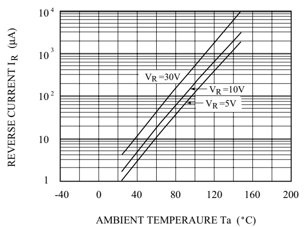
I_R - T_a
