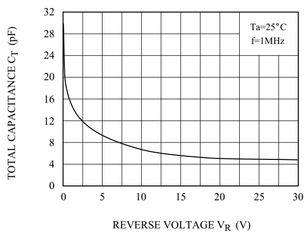
C_T - V_R
