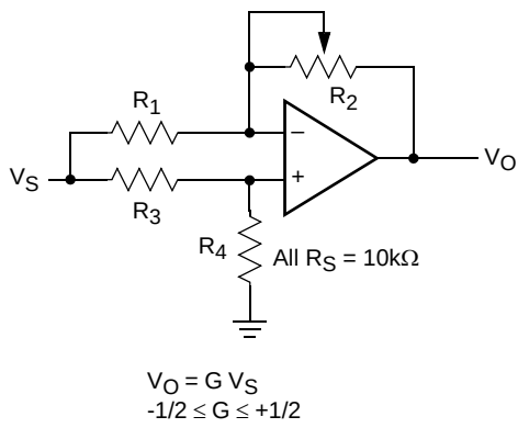
Attenuator
