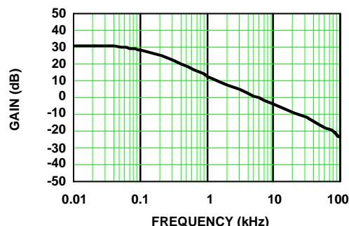
FIGURE 9A. GAIN
