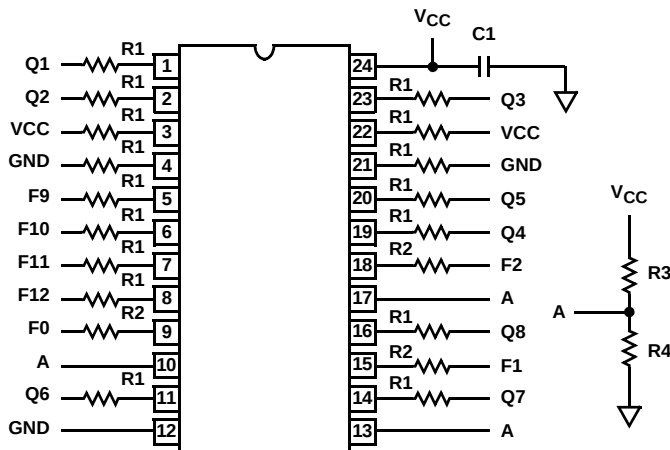
MD82C54 (CERDIP)
