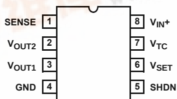
ICL7663S (PDIP, SOIC) TOP VIEW
