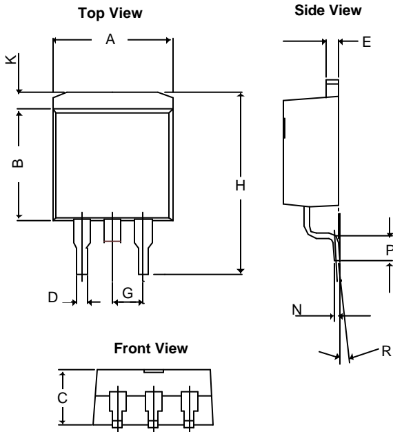
TO-263-2(D 2 PAK)
