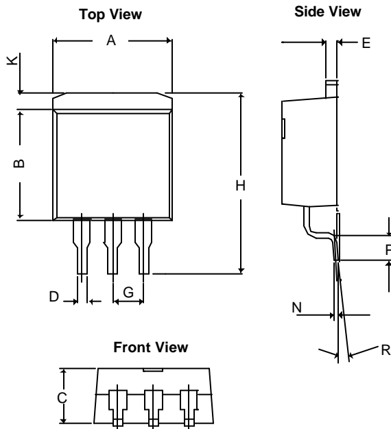
TO-263-3(D 2 PAK)
