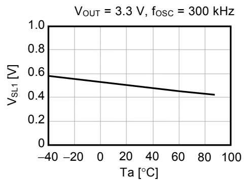
(10) \overline{\text{ON}}/\overline{\text{OFF}} 端子输入电压“L”1( V_{SL1} ) — 温度( T_a ) (11) \overline{\text{ON}}/\overline{\text{OFF}} 端子输入电压“L”2( V_{SL2} ) — 温度( T_a )
