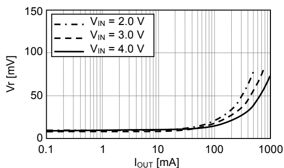
条件 4 S-8357B33
