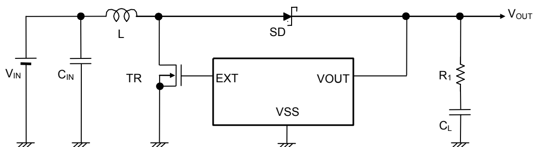
图27 陶瓷电容器使用电路示例
