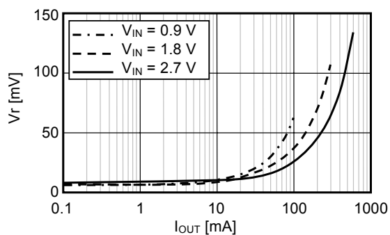
条件 11 S-8357F33
