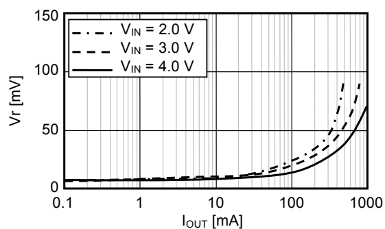
条件 5 S-8358B33
