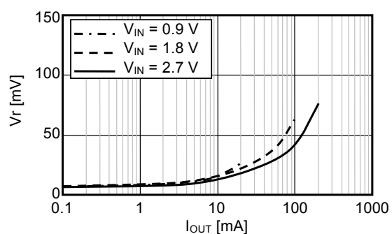
条件 13 S-8357N33
