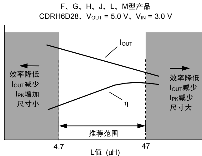
图 17 L 值— I_{OUT} 特性、L 值— \eta 特性
