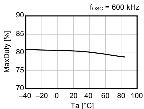
(8) PWM / PFM 切换占空系数(PFMDuty) — 温度( T_a ) (9) \overline{\text{ON}}/\overline{\text{OFF}} 端子输入电压“H”( V_{SH} ) — 温度( T_a ) (S-8356/58 系列)
