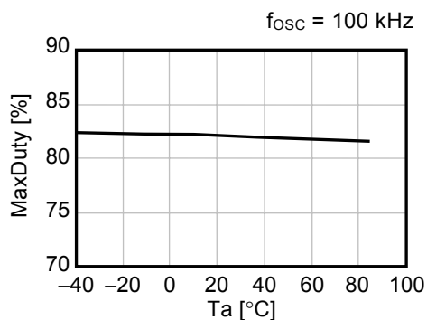
(7) 最大占空系数(MaxDuty) — 温度( T_a ) ( V_{OUT} = 3.3\text{ V} )
