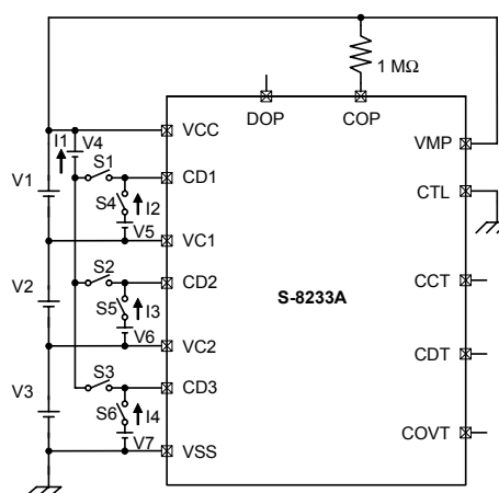
测定电路8
