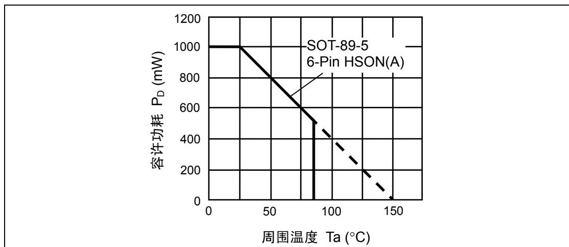
图4 封装容许功耗(线路板实际安装时)
