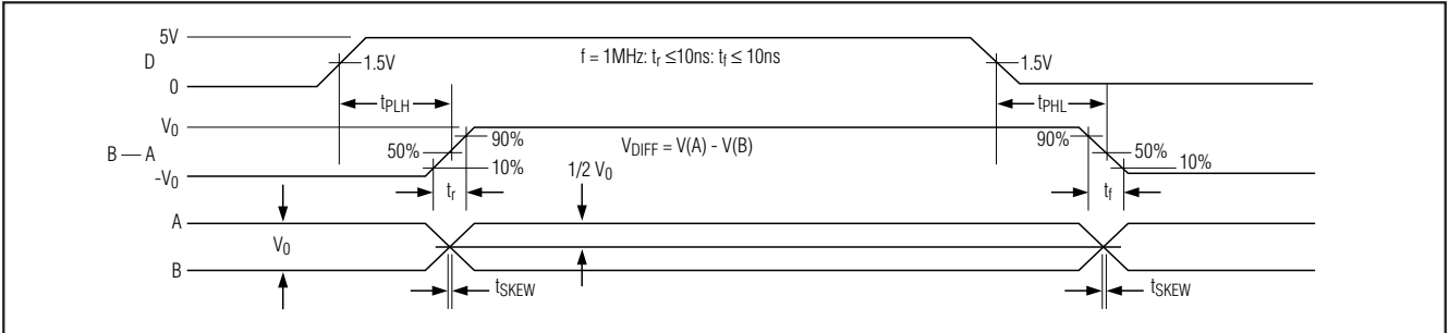
图 6. V.11、V.35 发送器传输延迟
