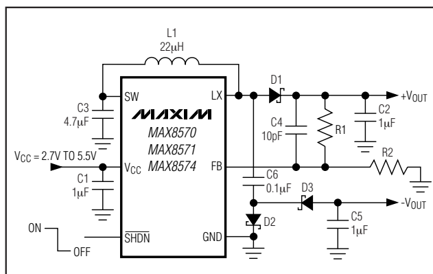
图5. 为LCD偏置提供负输出电压
