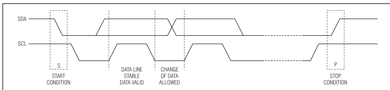
图5. I 2 C总线开始、停止和数据变化条件
