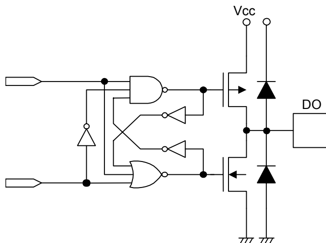
图23 DO端子
