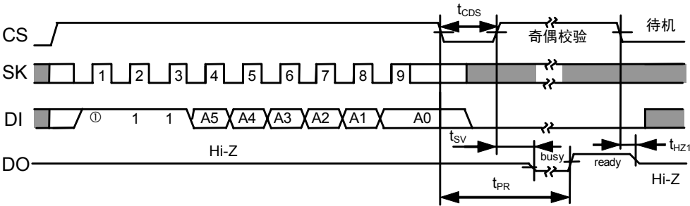
图 8 数据删除定时 (S-93A46A)
