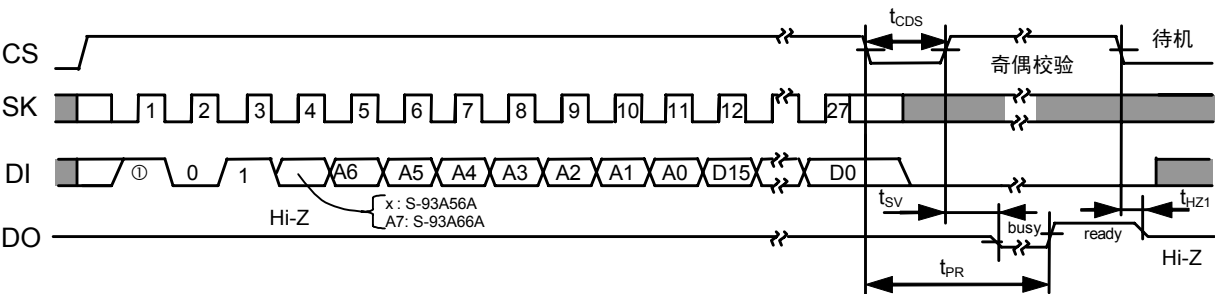
图7 数据写入定时 (S-93A56A, S-93A66A)
