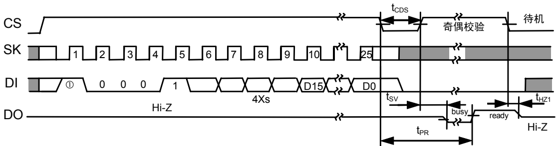
图10 全部写入定时 (S-93A46A)
