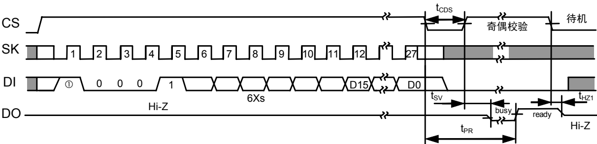
图11 全部写入定时 (S-93A56A, S-93A66A)
