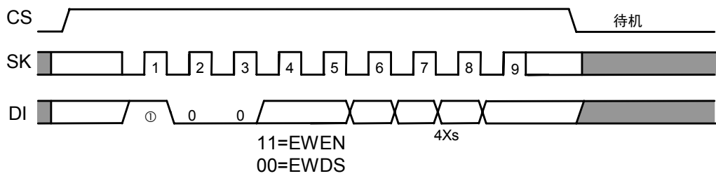
图14 写入允许 / 禁止定时 (S-93A46A)
