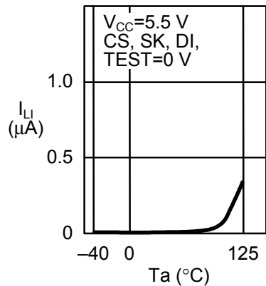
1.13 输入泄漏电流 I_{LI} —周围温度 T_a
