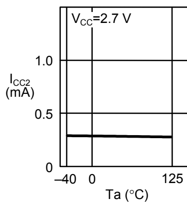
1.9 程序分析时消耗电流 I_{CC2} —周围温度 T_a
