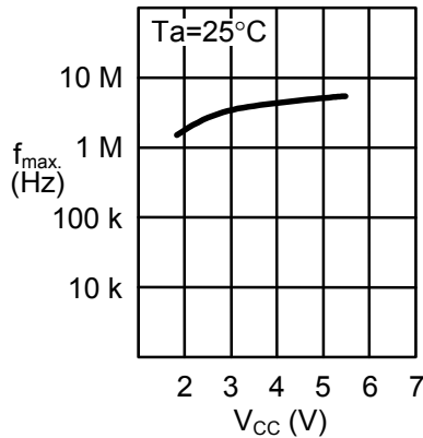
2.1 最大動作频率 f_{\max} —电源电压 V_{CC}
