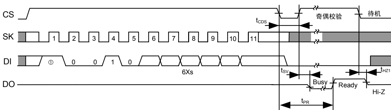
图13 全部删除定时 (S-93A56A, S-93A66A)
