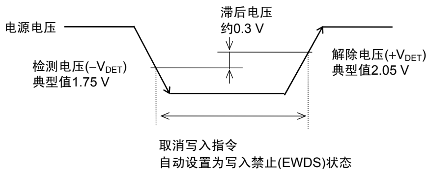
图16 低电源电压时的工作
