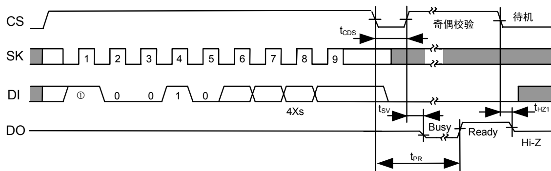
图12 全部删除定时 (S-93A46A)
