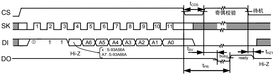
图 9 数据删除定时 (S-93A56A, S-93A66A)
