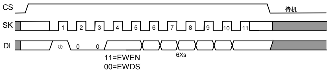
图15 写入允许 / 禁止定时 (S-93A56A, S-93A66A)
