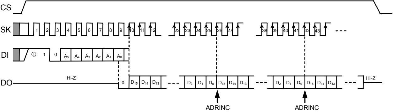
图4 读出定时 (S-93A46A)
