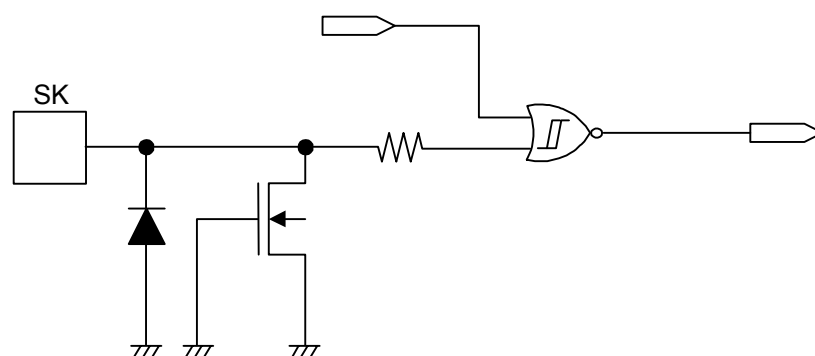
图20 SK端子
