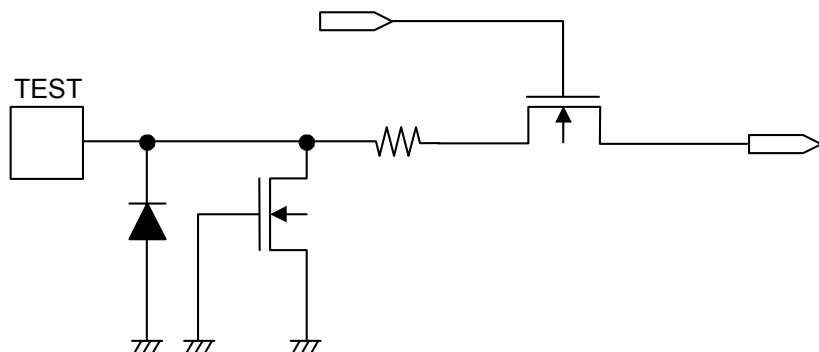
图22 TEST端子
