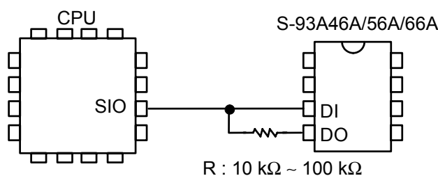
图18 3线式接口的连接法
