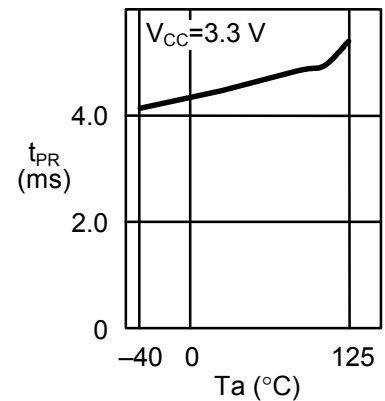
2.4 写入时间 t_{PR} —周围温度 T_a
