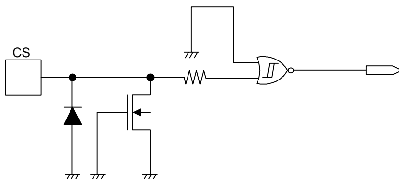
图19 CS端子
