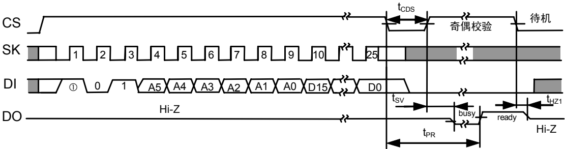
图6 数据写入定时 (S-93A46A)
