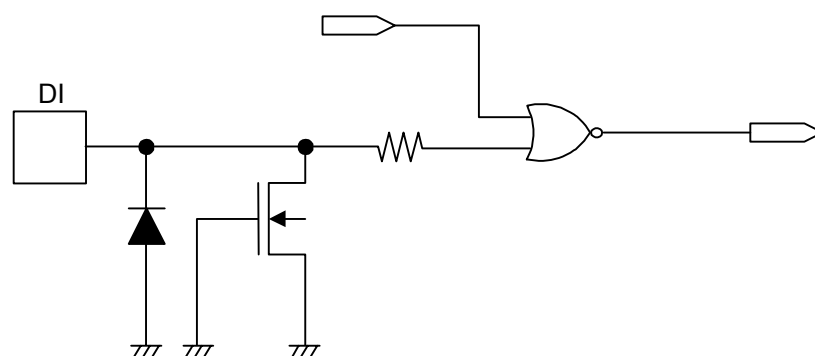
图21 DI端子
