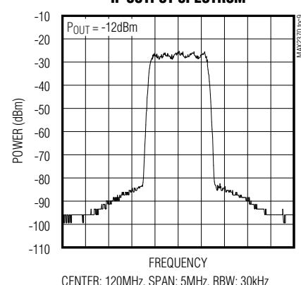
IF OUTPUT SPECTRUM
