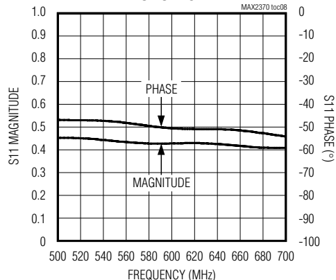
LO PORT S11
