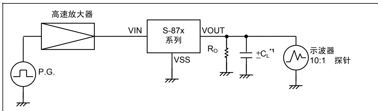
图 27 测定电路
