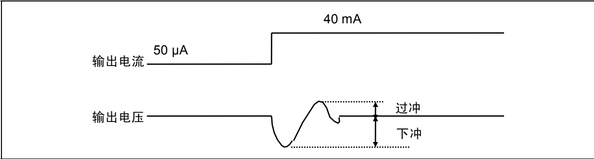
图 30 通过输出电流而引起输出电压的变动
