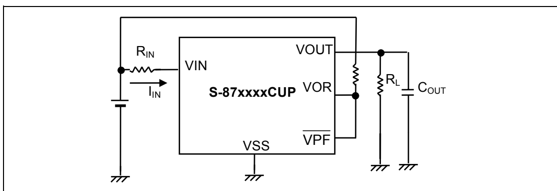
图 22 注意连接示例 1
