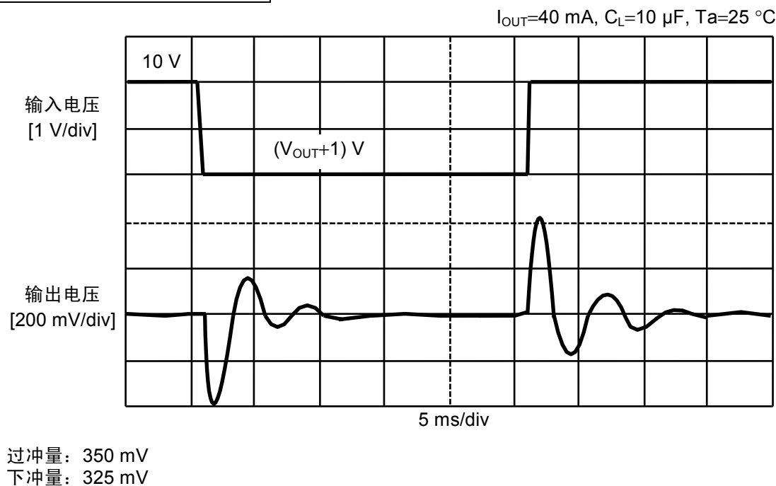
类型 1 ( (V_{OUT}+1) V \leftrightarrow 10 V 的矩形波)
