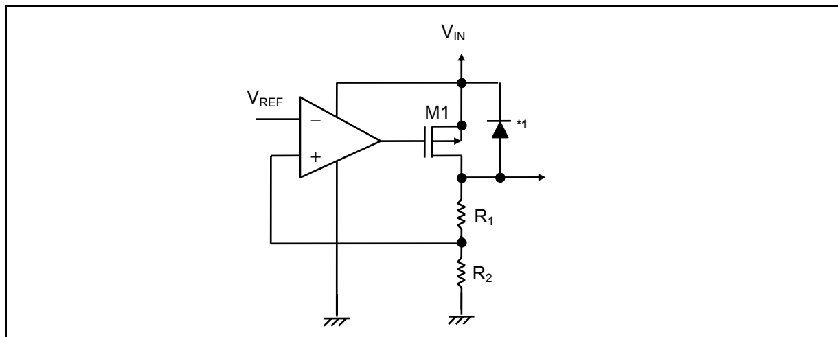
*1. 寄生二极管
