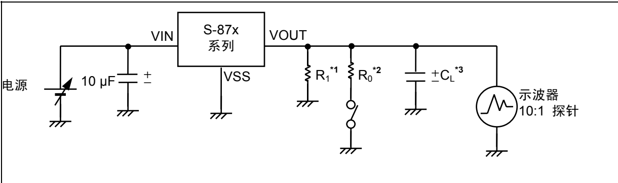
图 30 通过输出电流而引起输出电压的变动
