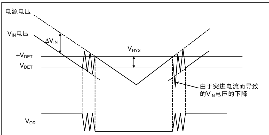
图 24 \Delta V_{IN} > V_{HYS} 时
