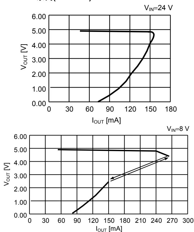
S-8750xxx 系列( T_a=25^\circ\text{C} )
