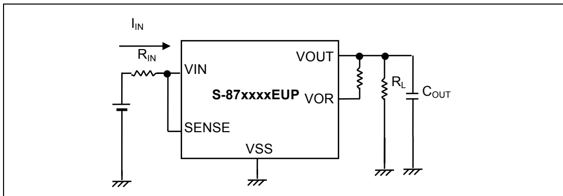
图 23 注意连接示例 2
