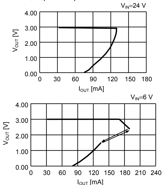
S-8730xxx 系列( T_a=25^\circ\text{C} )
