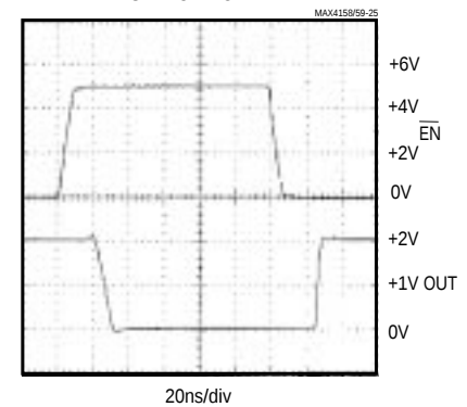
MAX4159/MAX4259 EN SWITCHING DELAY
