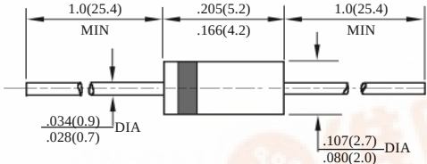
DO – 41
