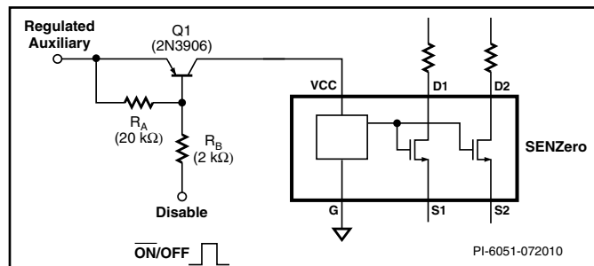
图 8. SENZero从稳压辅助绕组上电
