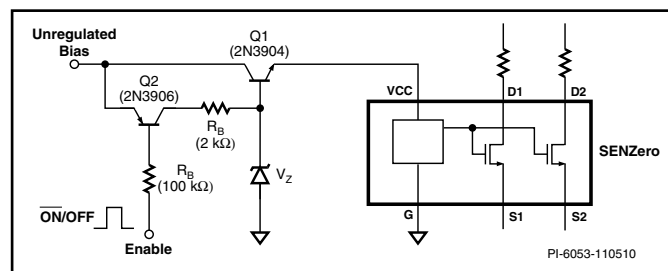
图 9. 非稳压偏置绕组通过串联稳压器上电的修改版电路。晶体管Q2提供远程关断功能
