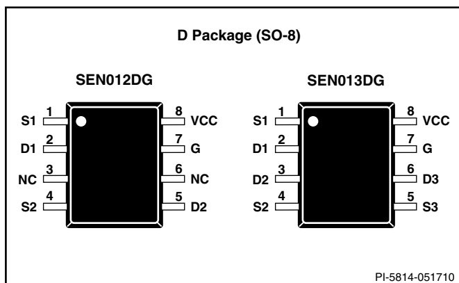
图 4. 引脚配置
