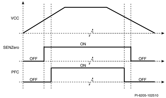
图 11. 在上电和断电期间，PFC IC与SENZero之间的时序。
