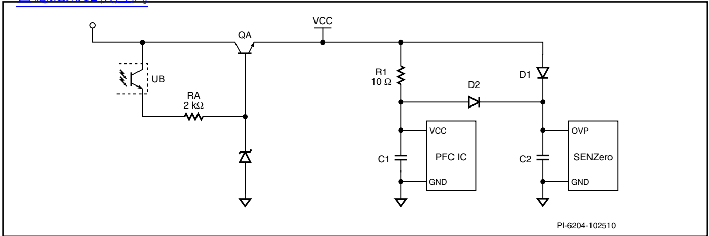
图 13. 出现 PS(ON) 信号时的典型连接
