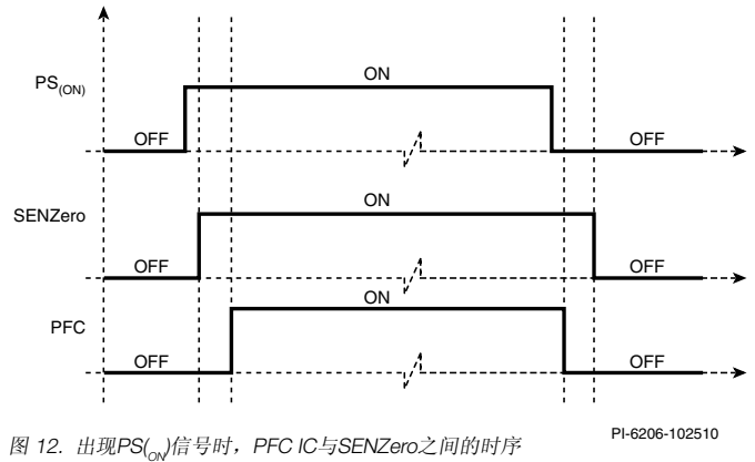
图 12. 出现PS (ON) 信号时，PFC IC与SENZero之间的时序
