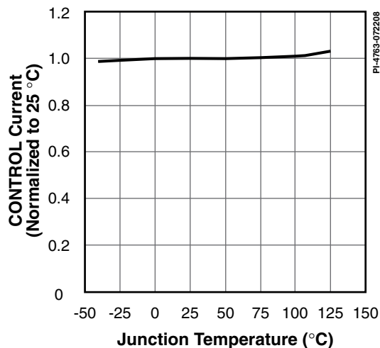
图 44. 占空比为0%时控制电流输出随温度的变化
