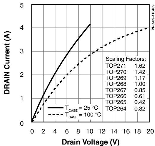
图 46. 输出特性
