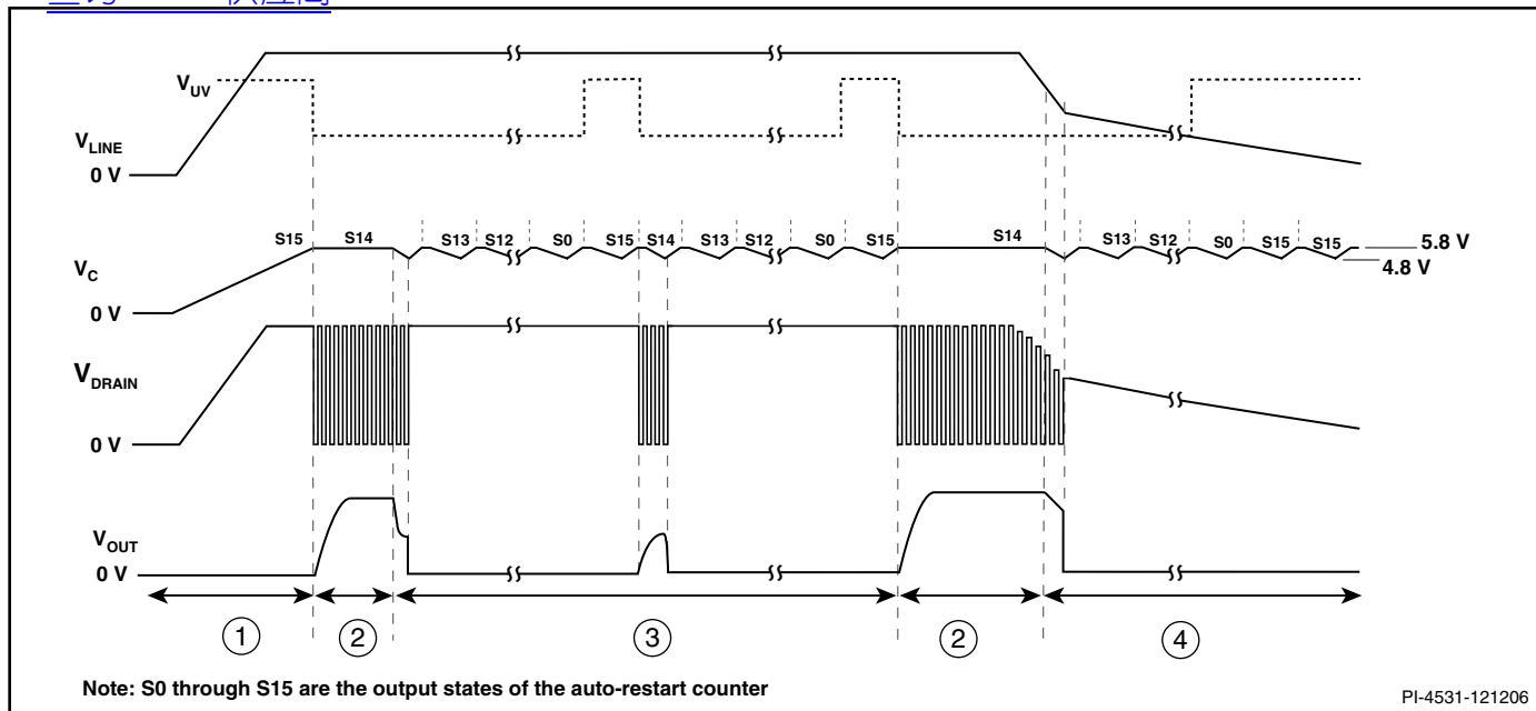
图 7. (1)上电(2)正常工作(3)自动重启动(4)电源关断时的典型波形
