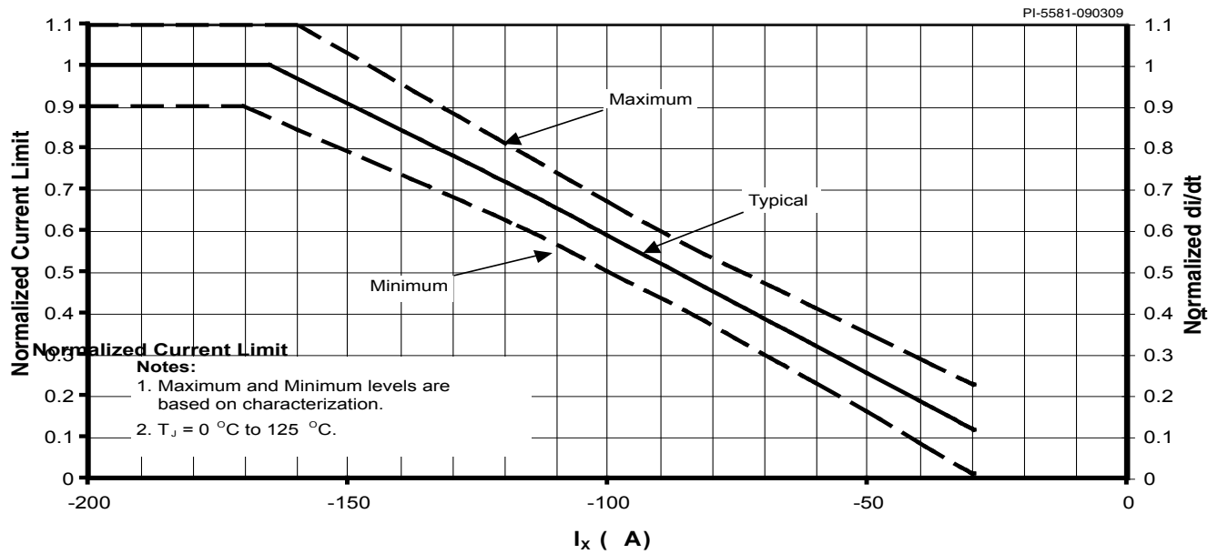
图 34. 归一化流限随X引脚电流的变化
