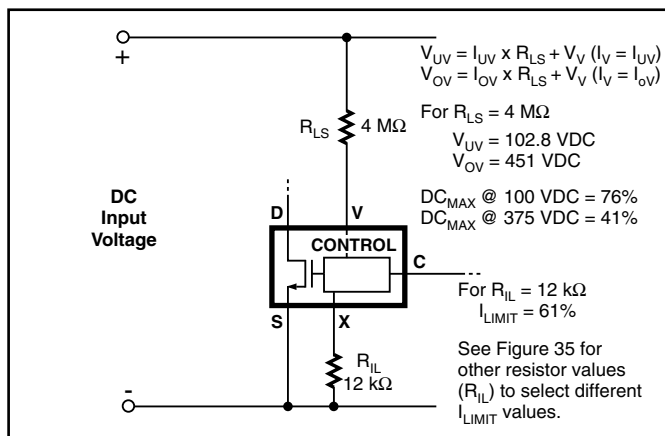
图 22. 线电压检测和外部设定流限
