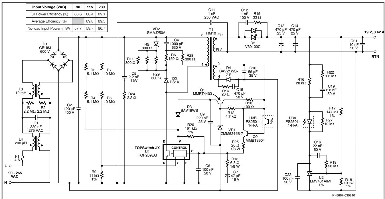
图 24. 低空载功耗、高效率的19 V, 65 W通用输入适配器电源
