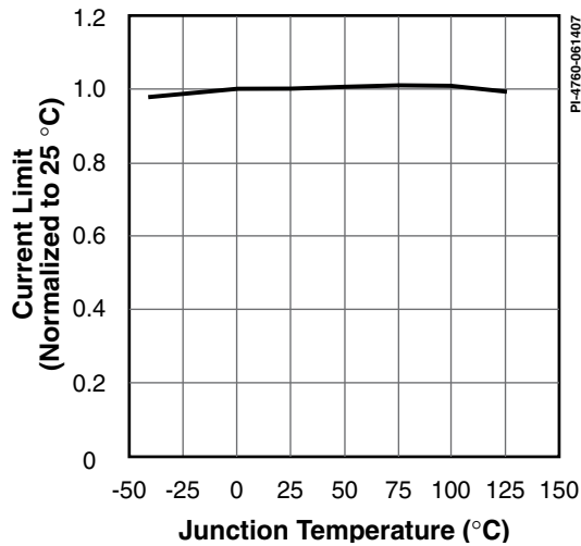
图 38. 内部流限随温度的变化
