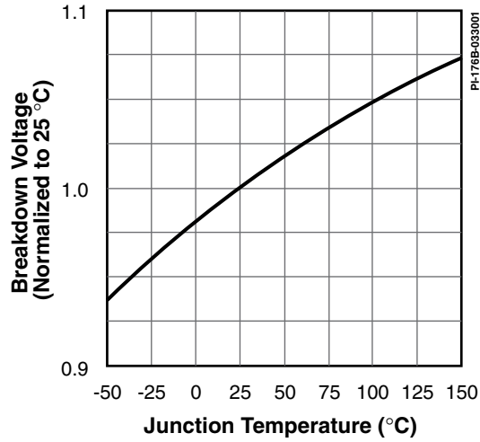
图 36. 击穿电压随温度的变化
