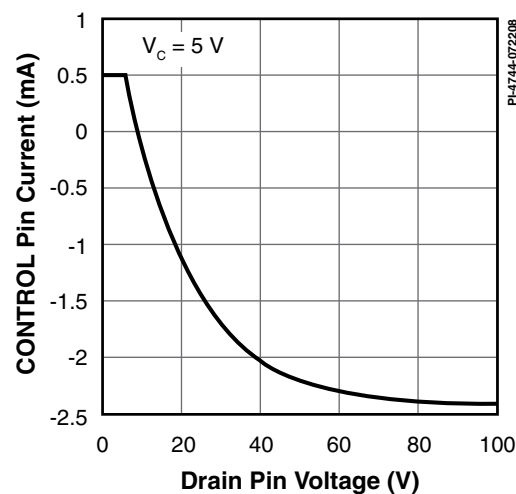
图 47. I_C 随漏极电压的变化
