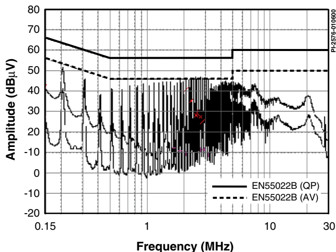
图 26. 不带抖动的固定频率工作
