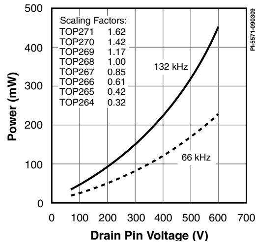
图 49. 漏极电容功耗
