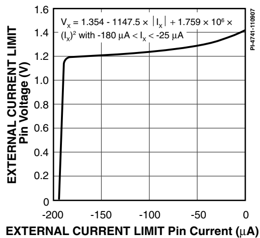
图 43. 外部流限引脚电压随电流的变化
