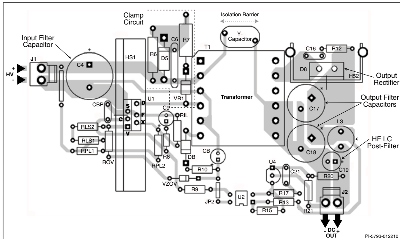
图 29. 使用E封装、工作频率为132 KHz的TOPSwitch-JX的布板考量
