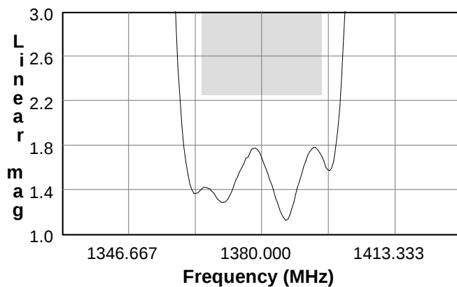
S11 VSWR
