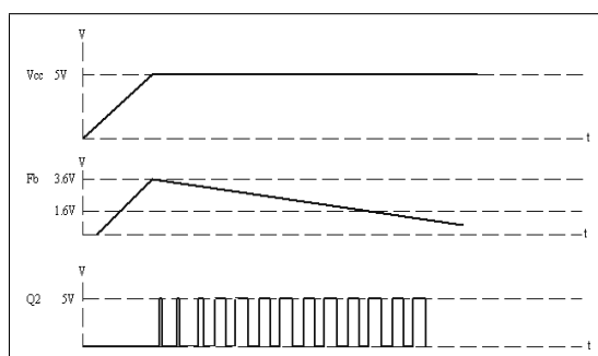
上电时序图
