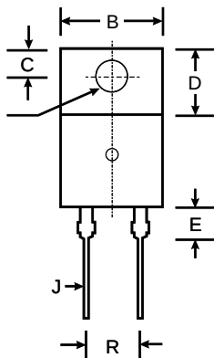
TO-220AC-P
