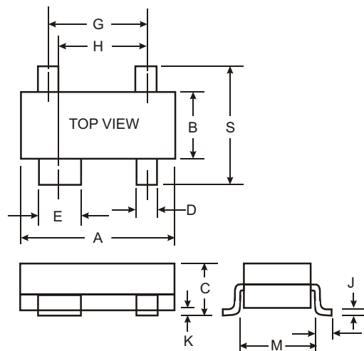
SOT-343 / SOT-143
