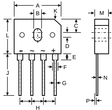
GBU
