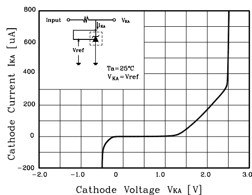
Fig. 5 I_{MIN} vs. V_{KA}
